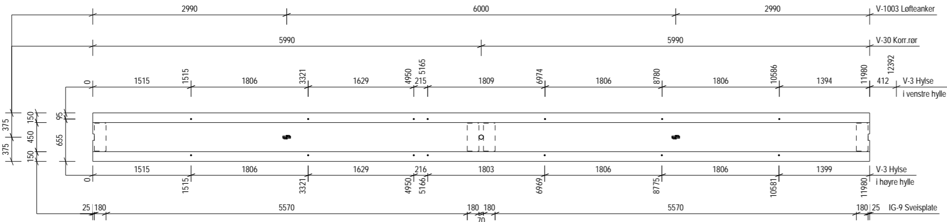
INNSTØPINGSGODS Sett fra overside form
