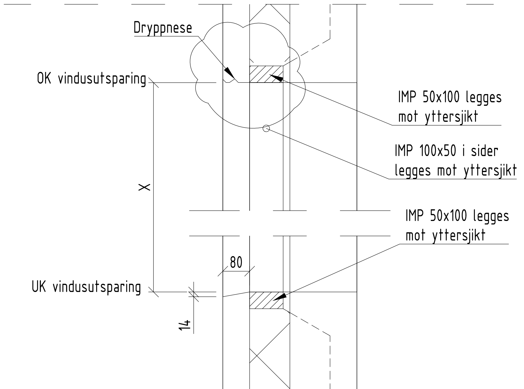
Detalj vindusutsparing
