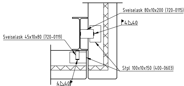
c) INNFESTING MOT I STÅLSØYLE
