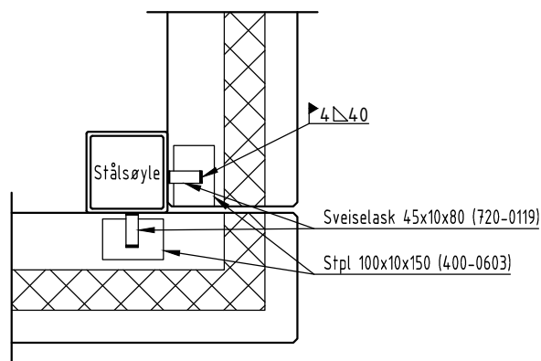
b) INNFESTING MOT HUP STÅLSØYLE
