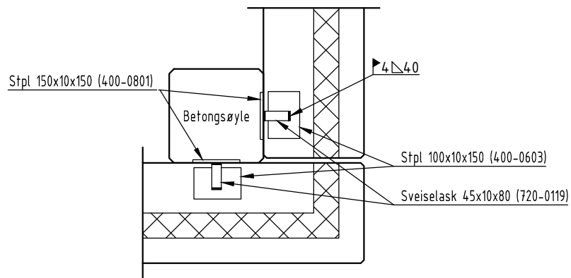
a) INNFESTING MOT BETONGSØYLE
